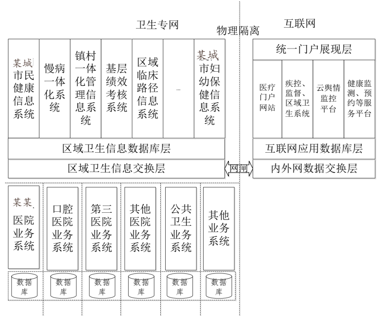
系统逻辑架构
